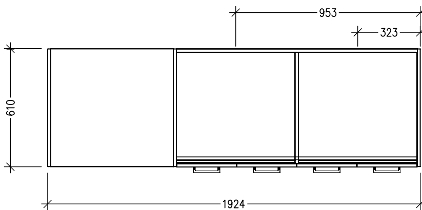
TOP VI
